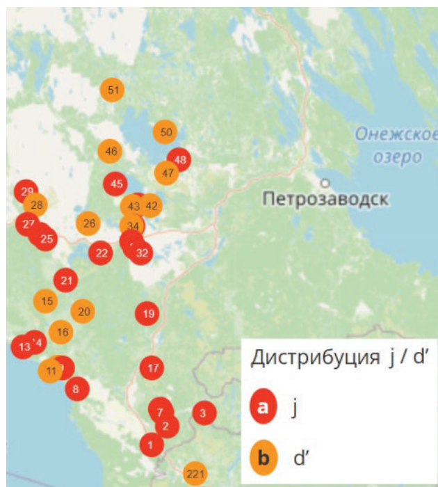
Рис. 5. Рефлексы *j
