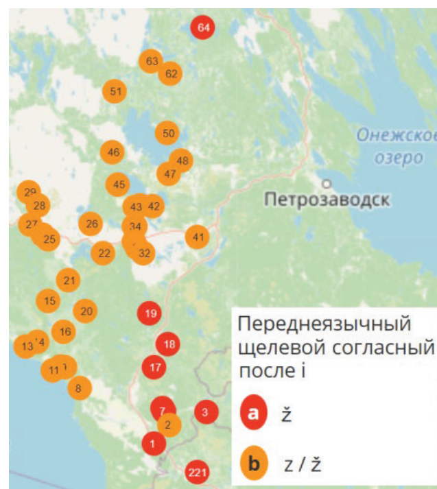
Рис. 4. Рефлексы *is
