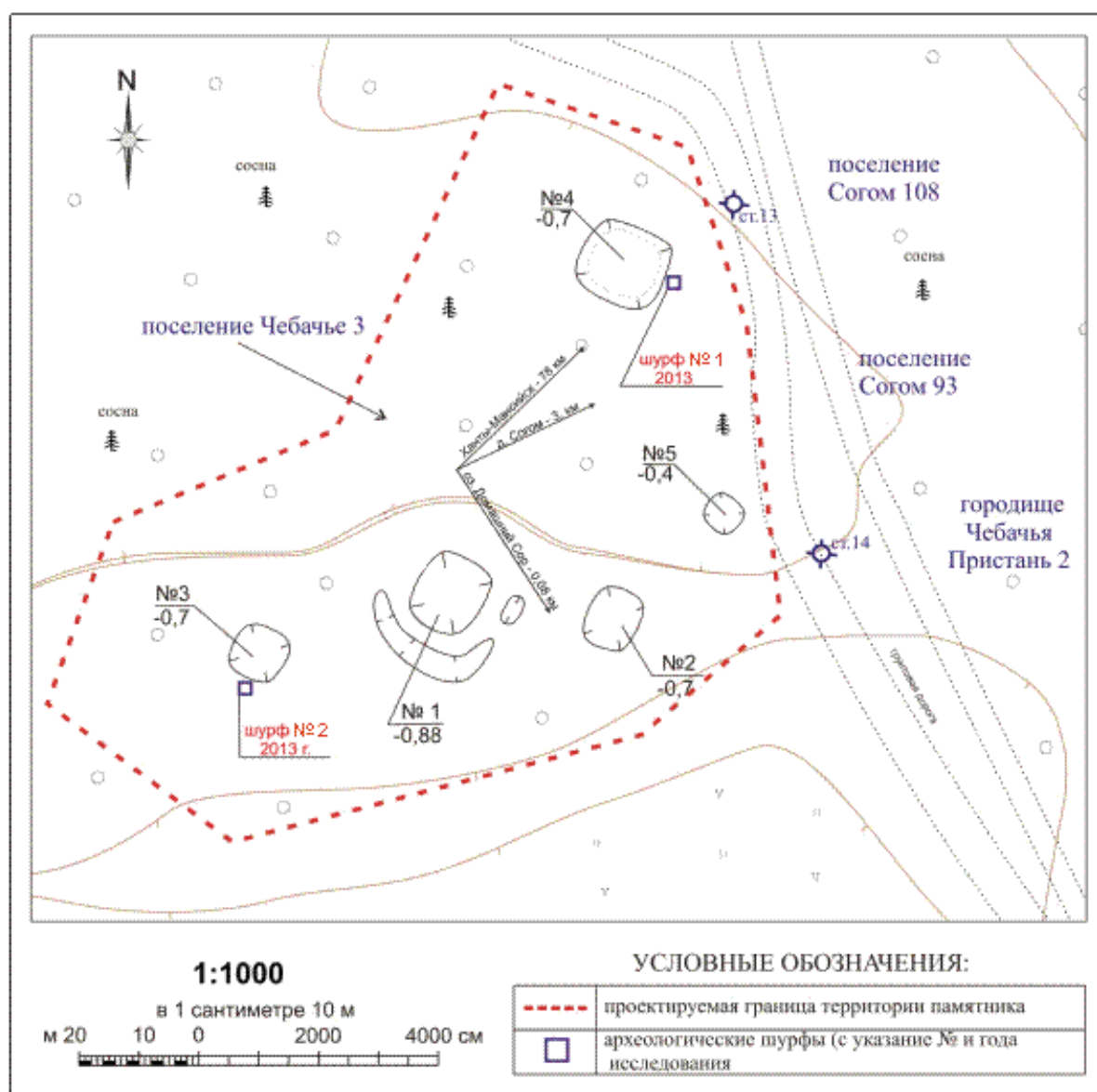
Рис. 1. План поселения Чебачье 3
