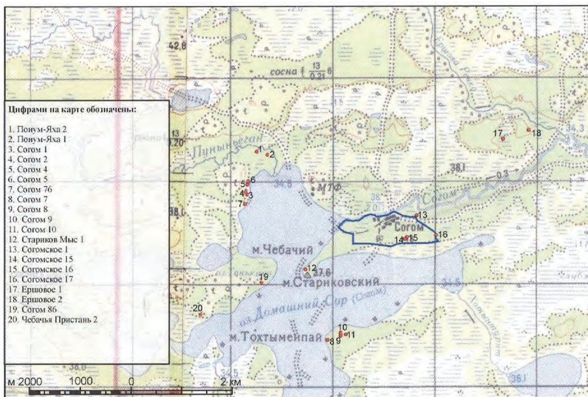
Рис. 1. Карта-схема расположения средневековых городищ Согомского археологического микрорайона.
